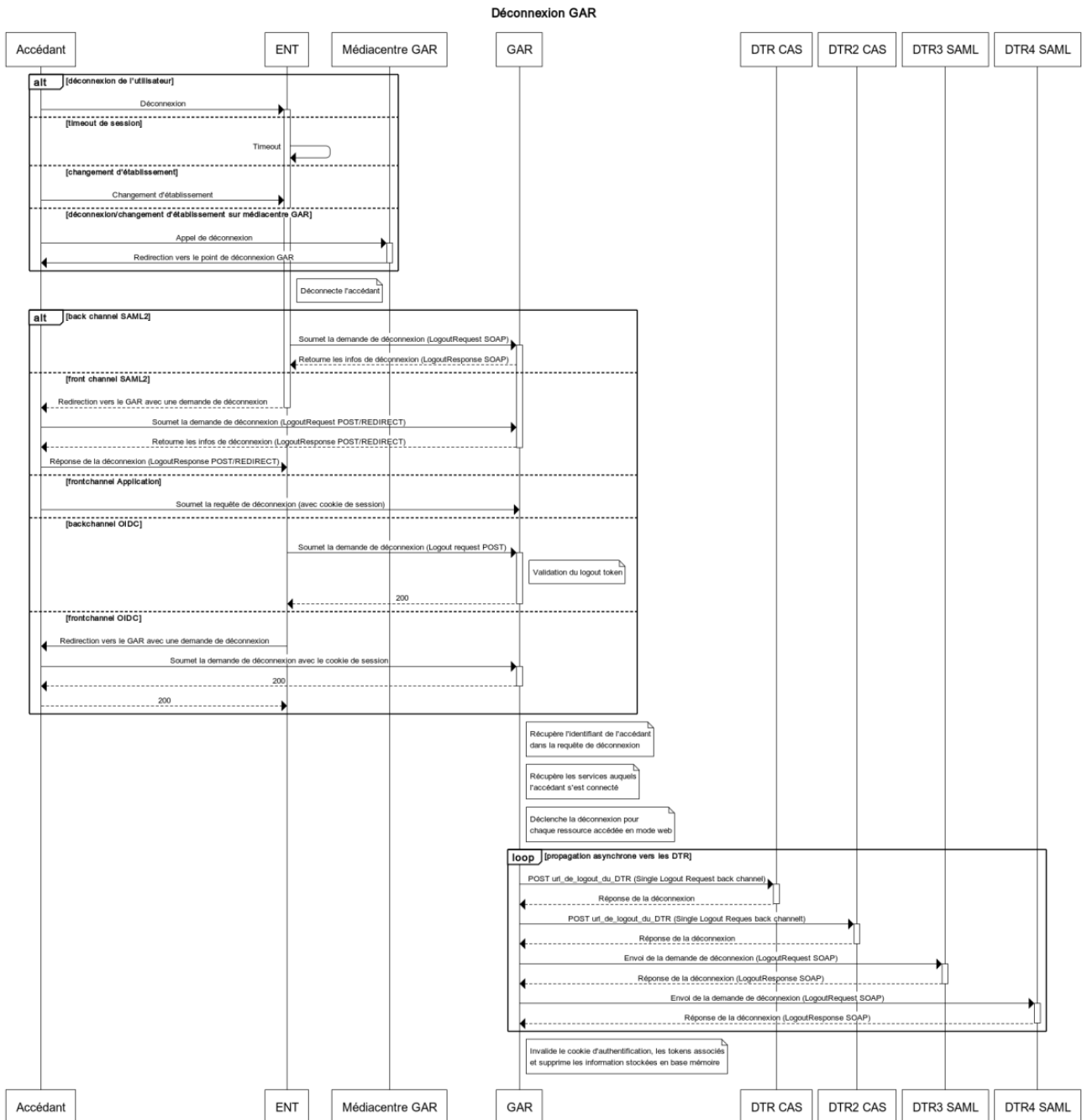
Figure 21 - Diagramme de séquence de la propagation de la déconnexion aux ressources
