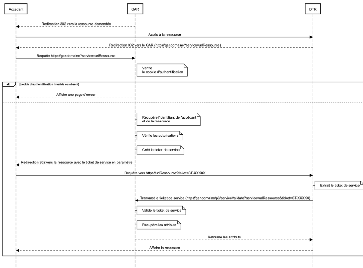
Figure 20 - Diagramme de séquence d'un accès CAS 3.0 ou supérieur à une ressource
