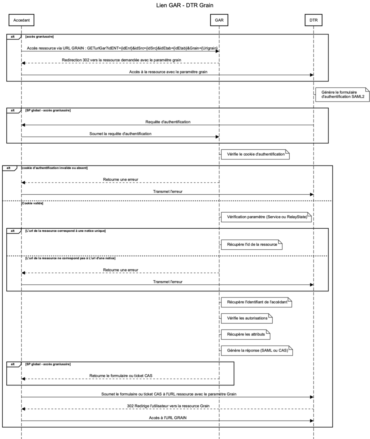
Figure 22 - Diagramme de séquence pour l'accès à un grain
