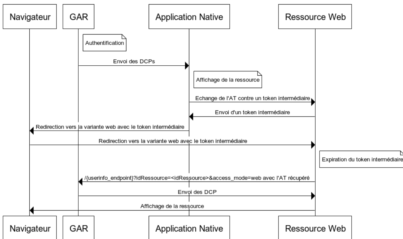
Figure 9 - Accès web par l'intermédiaire d'un Access Token
