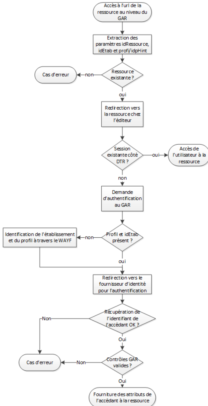
Figure 18 - Diagramme d'authentification par le GAR d'un utilisateur à une ressource
