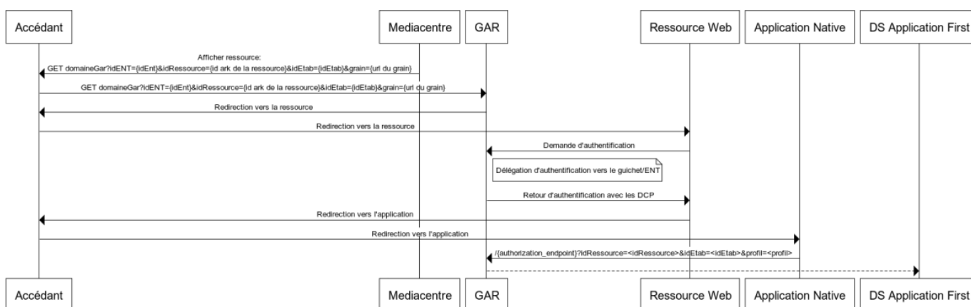
Figure 7 - Accès depuis le médiacentre avec une session GAR ouverte
