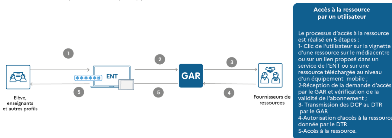
Figure 17 - Module d'accès aux ressources – accès web
