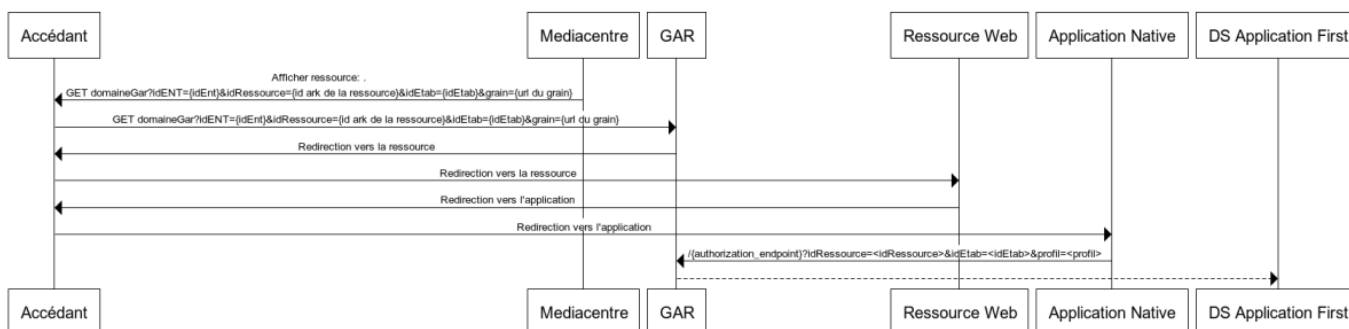
Figure 6 - Accès depuis le médiacentre sans session GAR ouverte
