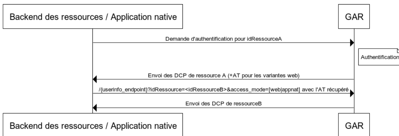
Figure 11 - Récupération des DCP pour deux ressource d'une même plateforme DTR
